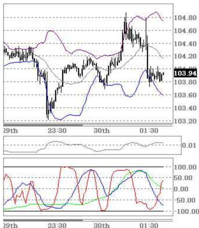
USD/JPY 30分足
